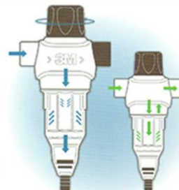
反沖洗水流方向 日常工作水流方向
